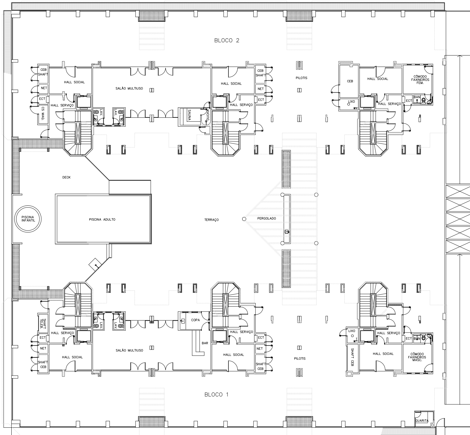
PLANTA BAIXA_ ORIGINAL ESC: 1/250
