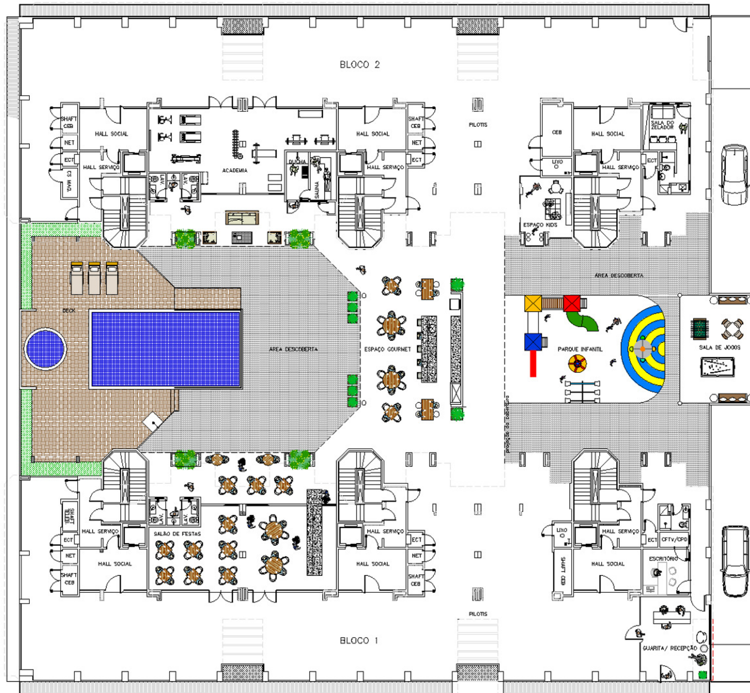
PLANTA BAIXA_ OPÇÃO 01 ESC: 1/250
